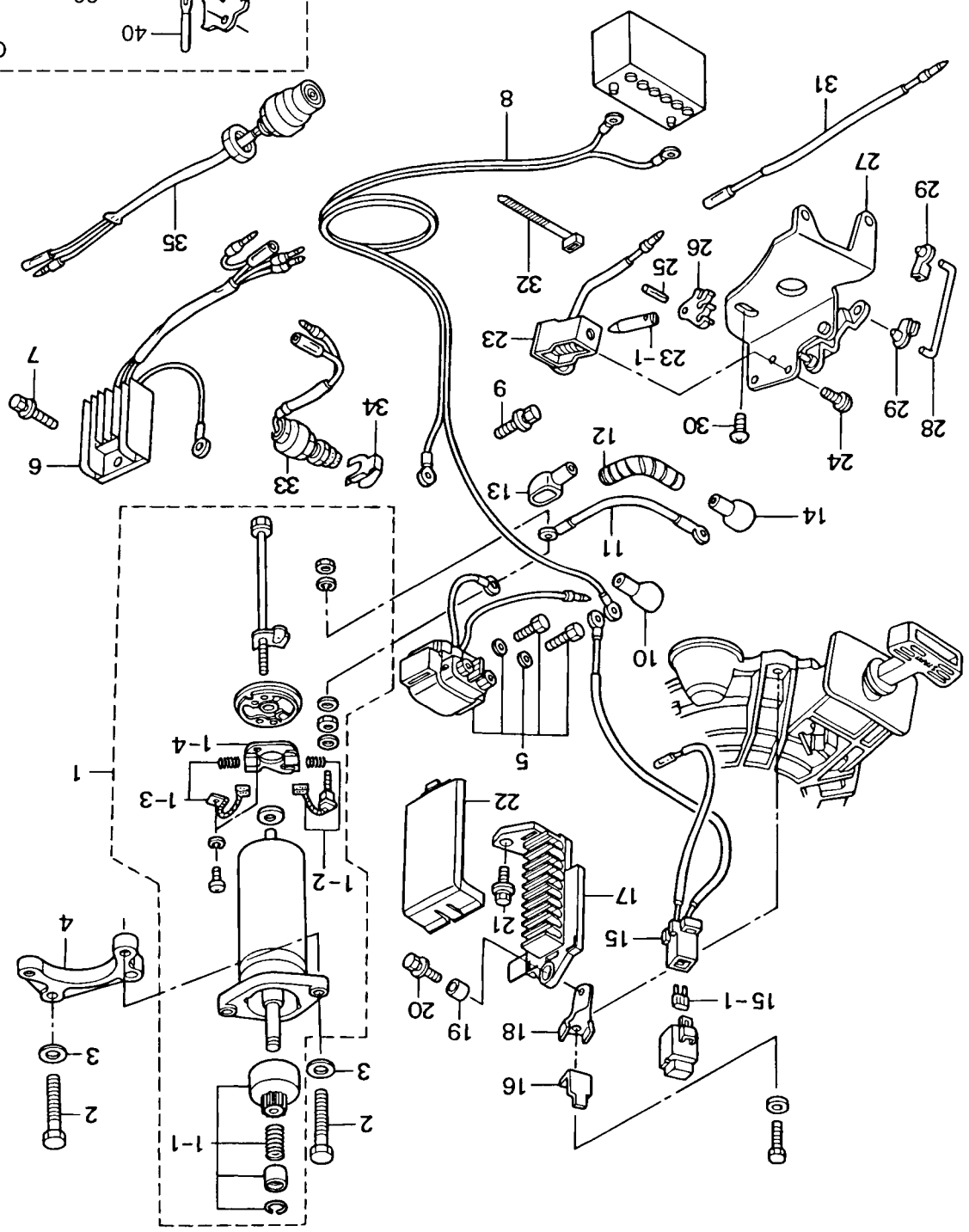
Fig. 9 ELECTRIC PARTS 電気部品
