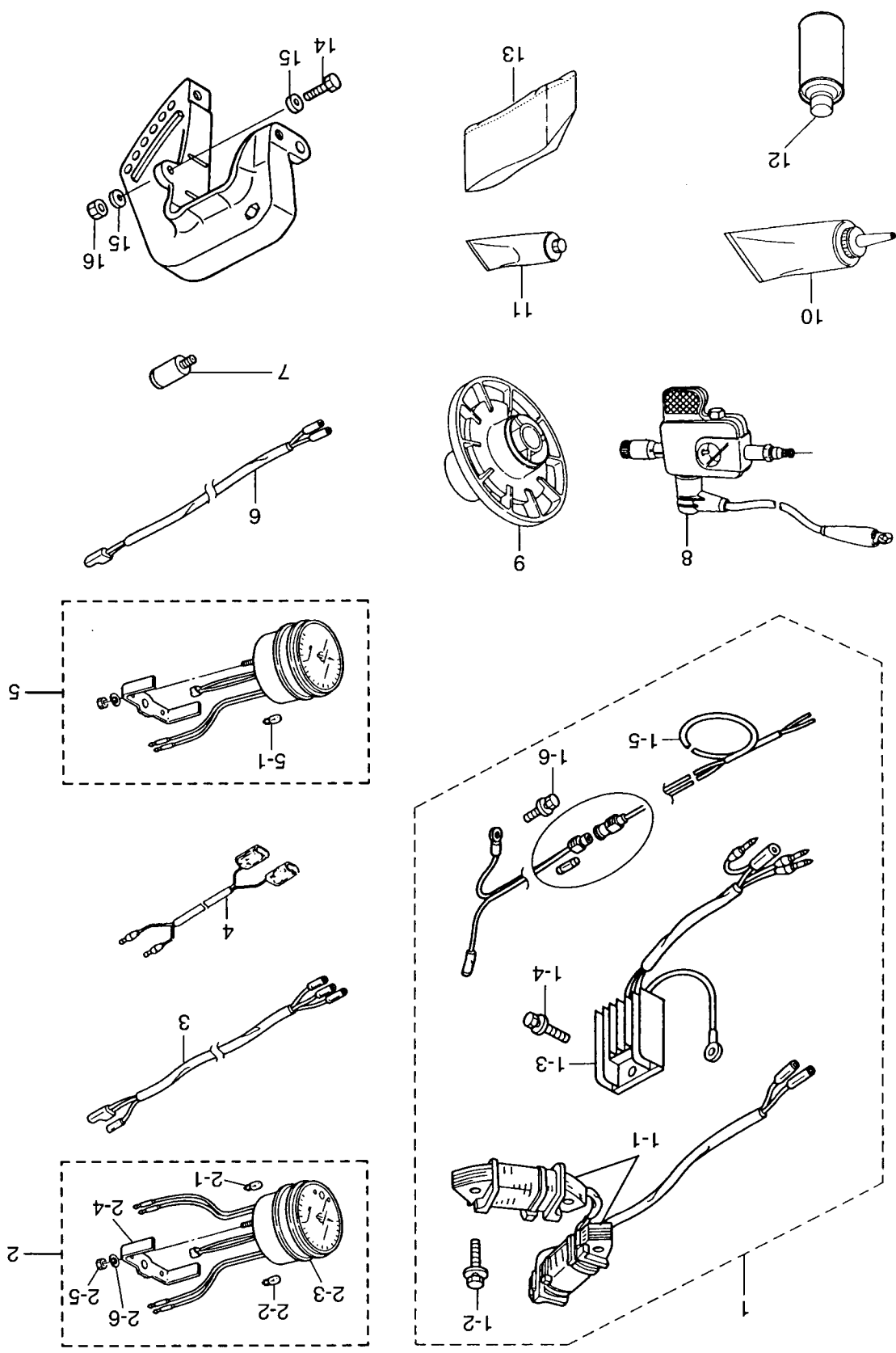
Fig. 21 OPTIONAL PARTS (ACCESSORIES) オプションパーツ (アクセサリ)
